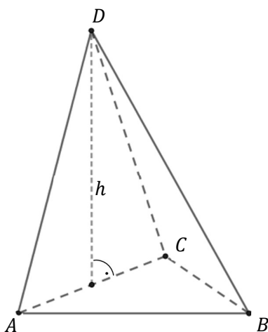
Kąt między krawędzią BD , a podstawą ostrosłupa.
